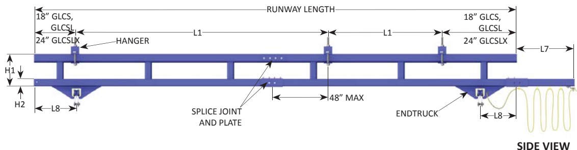
GLCS, GLCSL, GLCSLX STEEL RUNWAY
